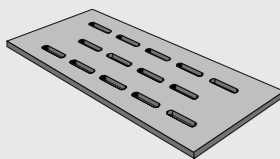
Pool Grid Type A Rejilla Piscina Tipo A 298x898x20 mm. 298x1198x20 mm.
